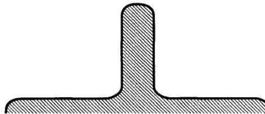
Рисунок Д.2 Форма сварных швов и обработка щелей
