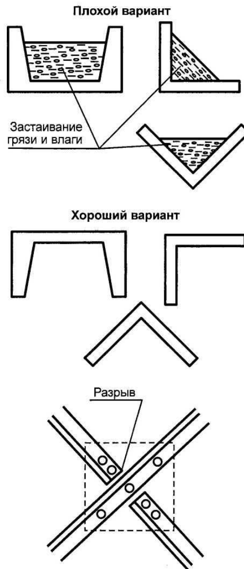
Рисунок Д.1 Исключение образования мест скопления влаги и грязи
